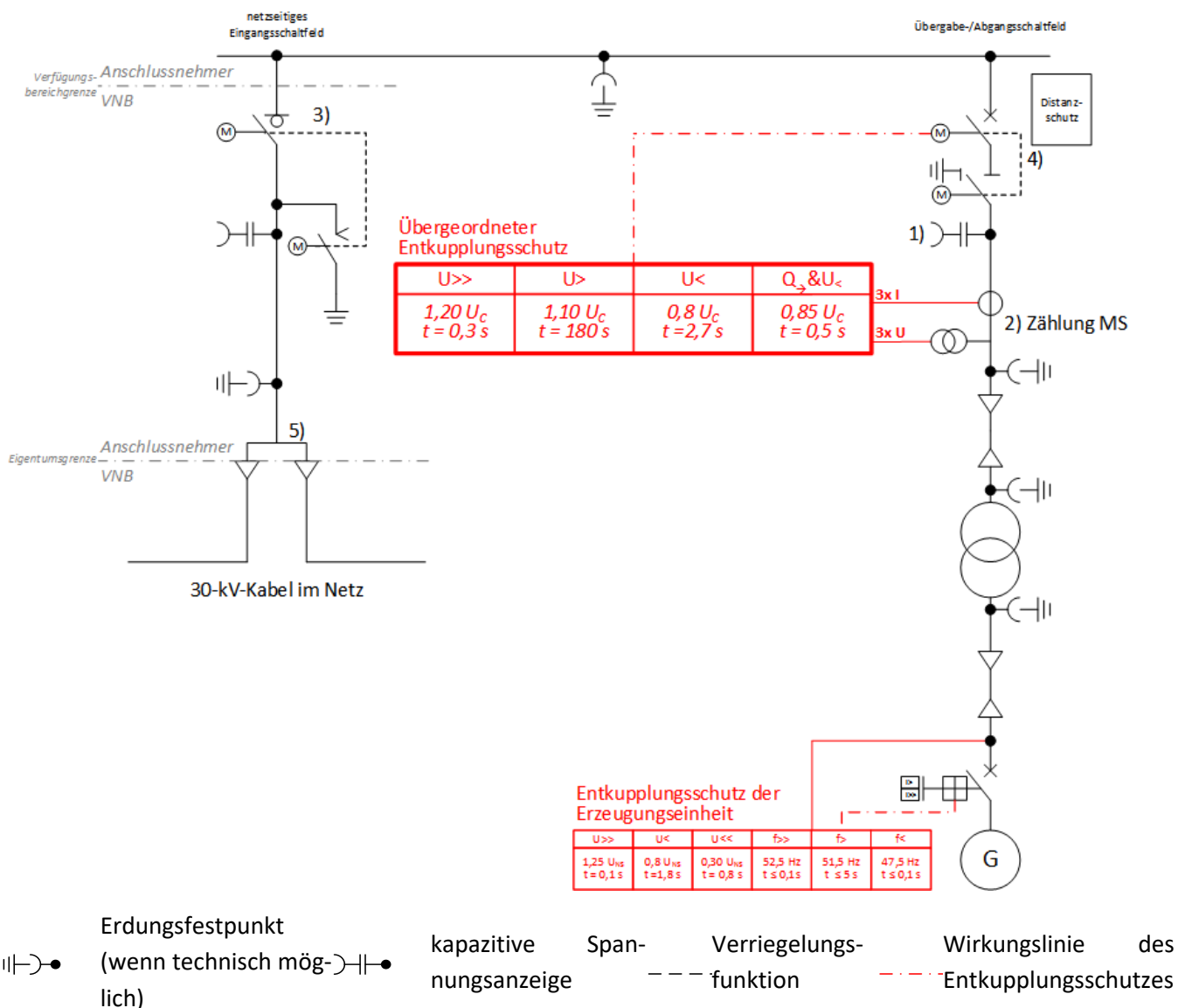
Bild D6: 35-kV-Anbindung einer Erzeugungsanlage im Netz
