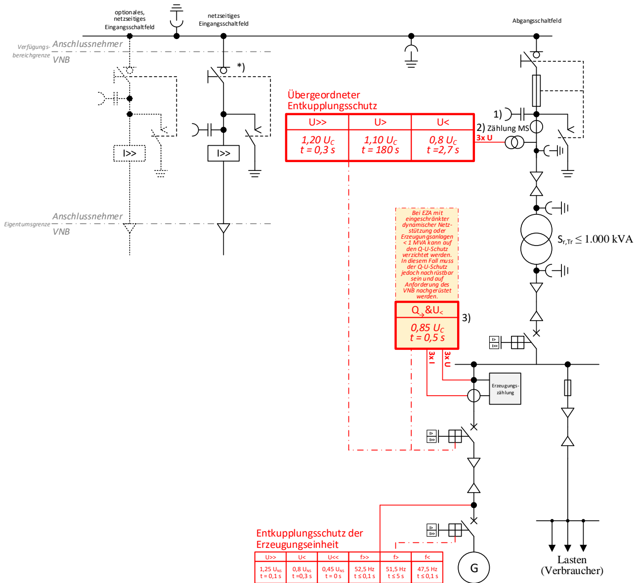
Bild D5a: 10 (20)-kV-Anbindung einer Mischanlage über einen Transformator
